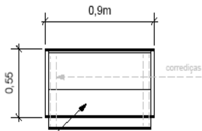
TECLADO RETRÁTIL COM CORREDIÇAS TELESÓPICAS
