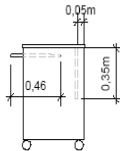
VISTA LATERAL
