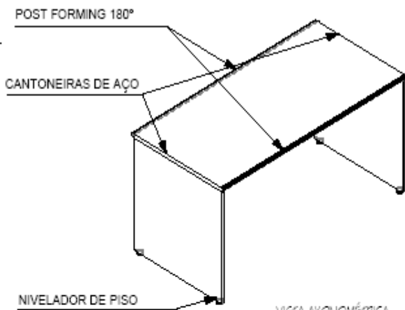
VISTA AXONOMÉTRICA
